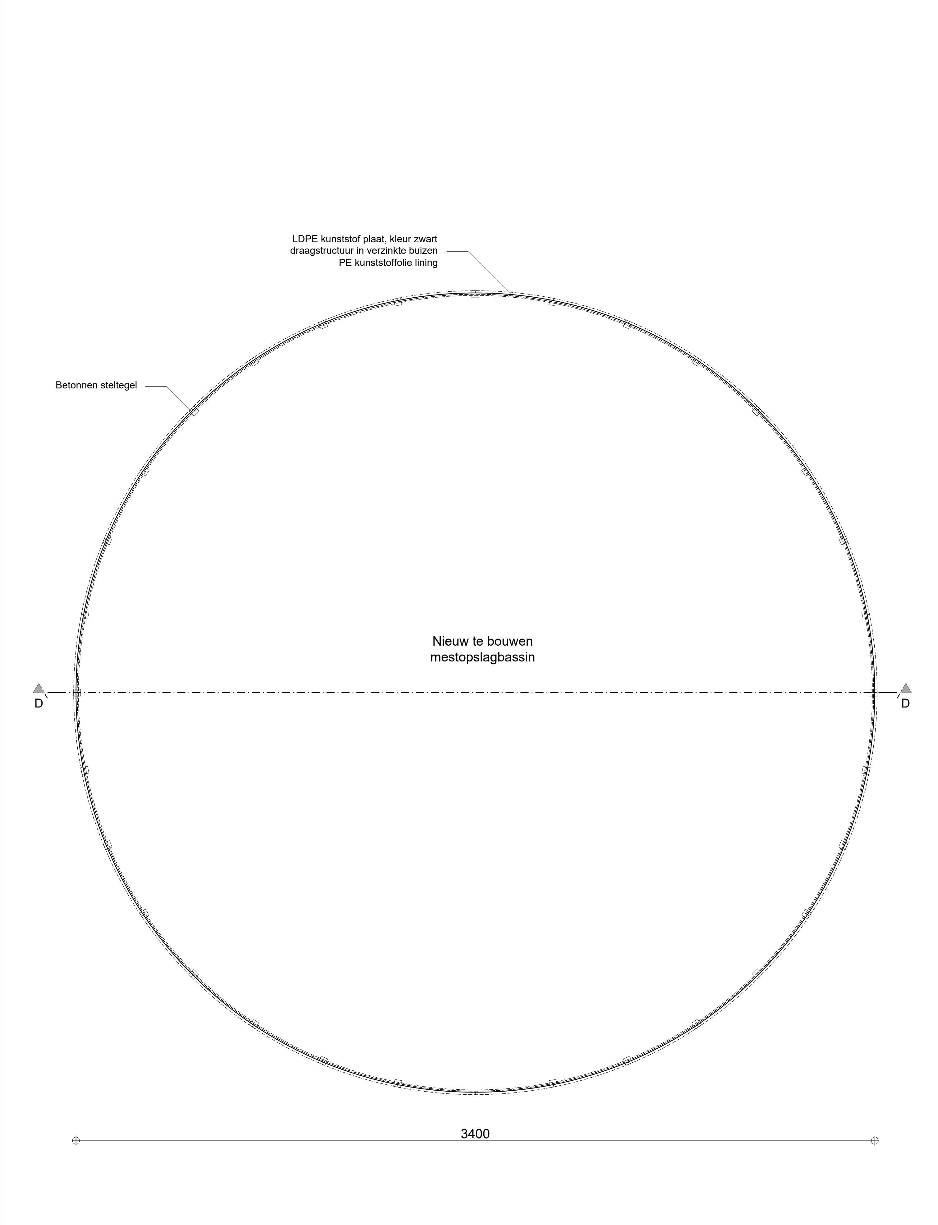
Mestbassin Grondplan 1/100 0 100 200 Gewenste toestand
