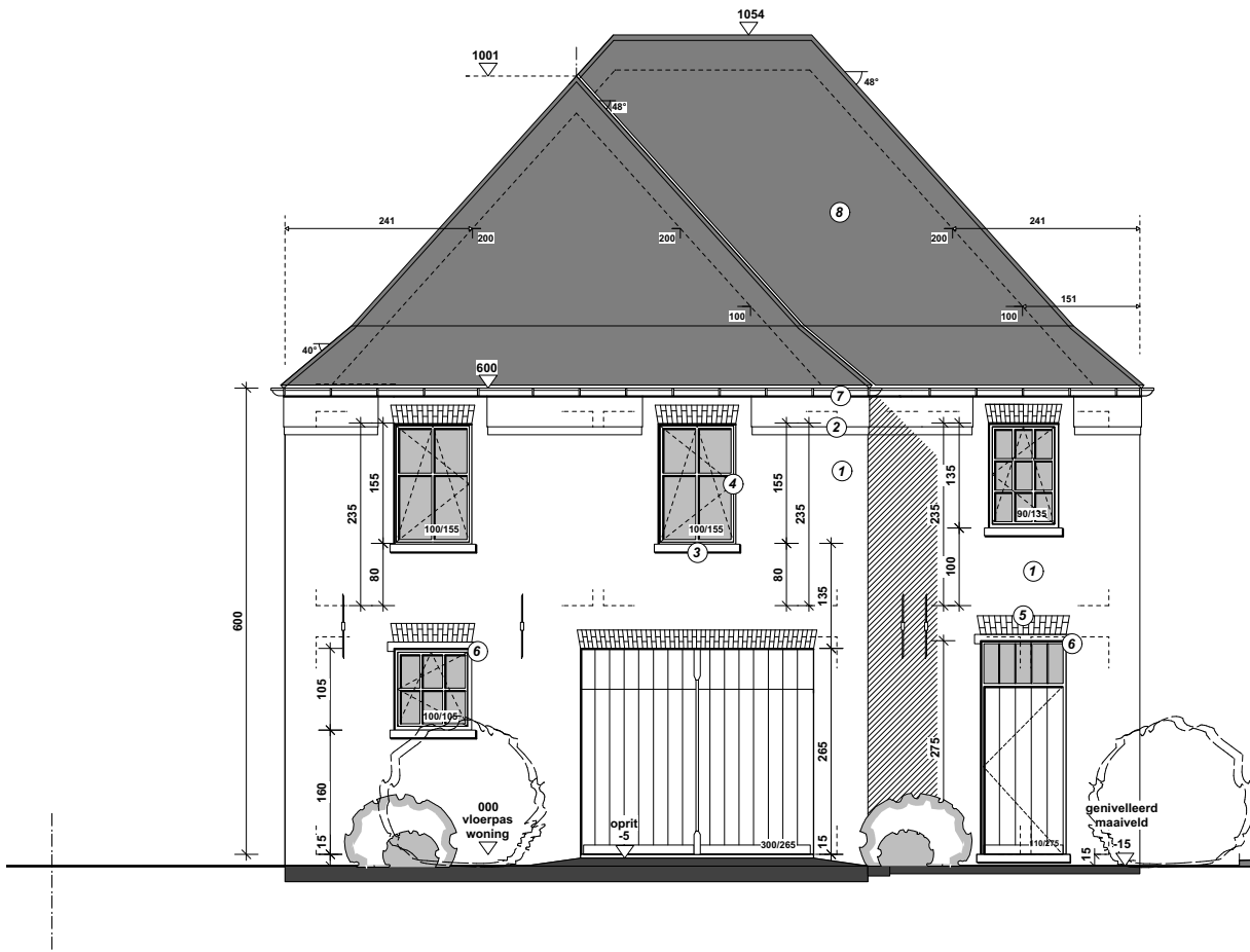
VOORGEVEL 1/100
