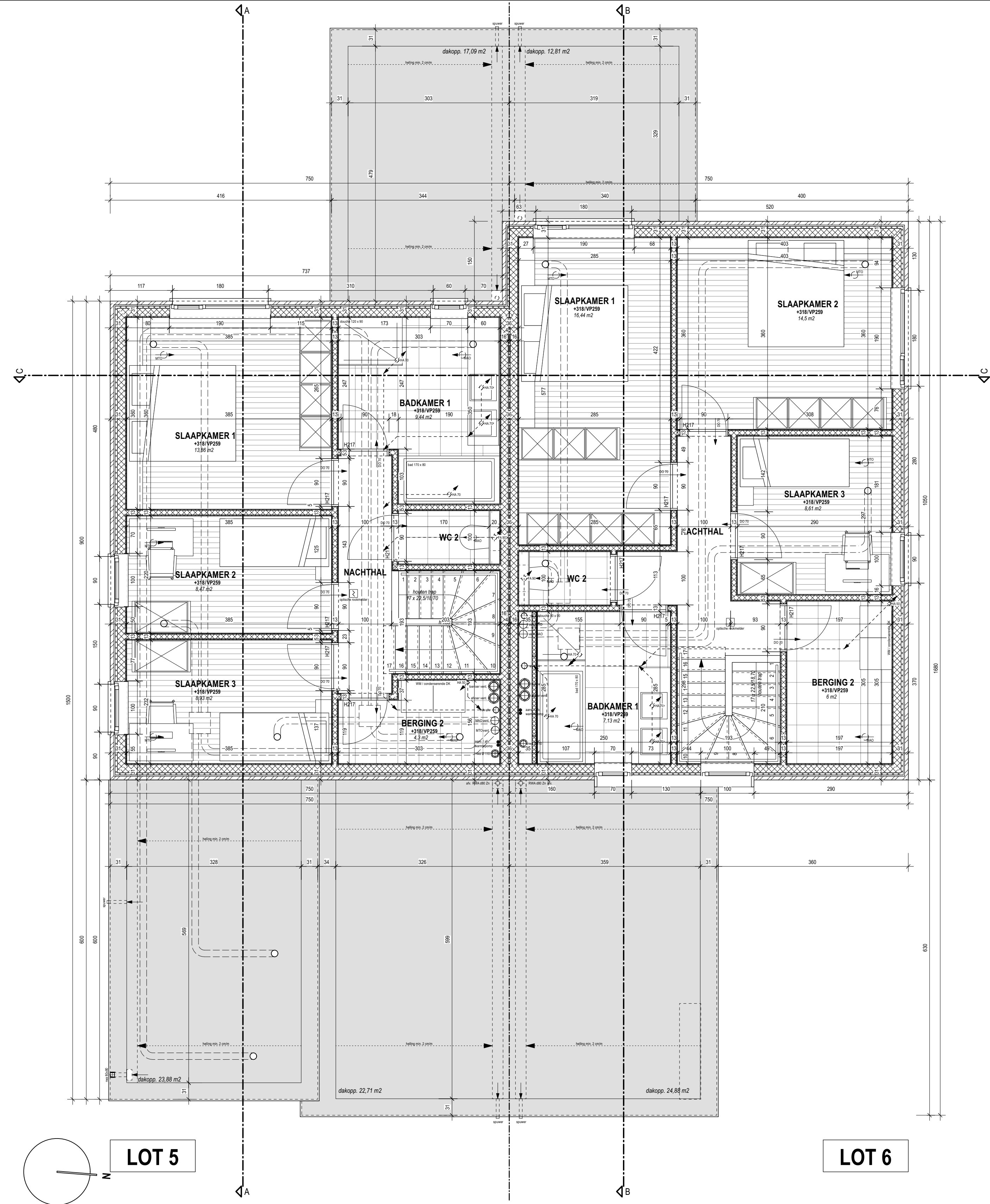
GRONDPLAN VERDIEPING +01 - nieuwe toestand | 1:50
