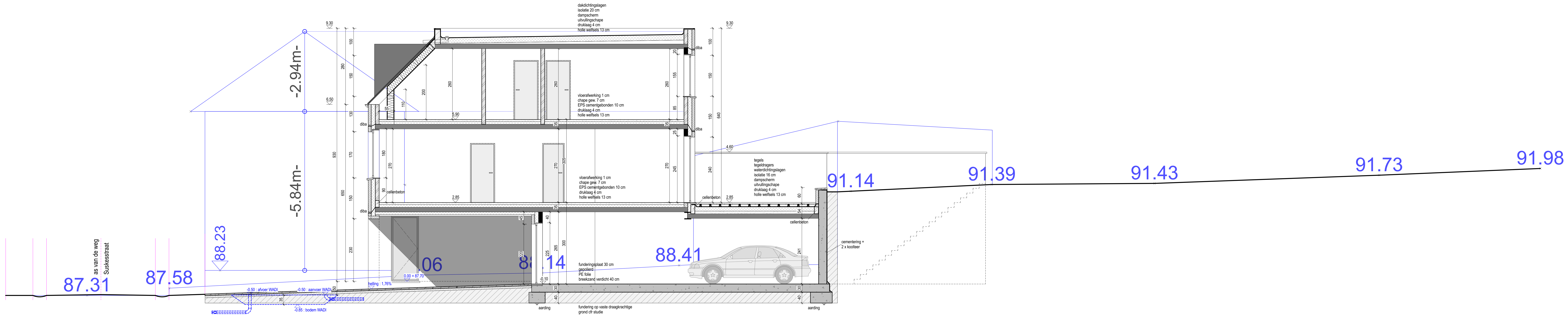
DOORSNEDE A-B 1/50
