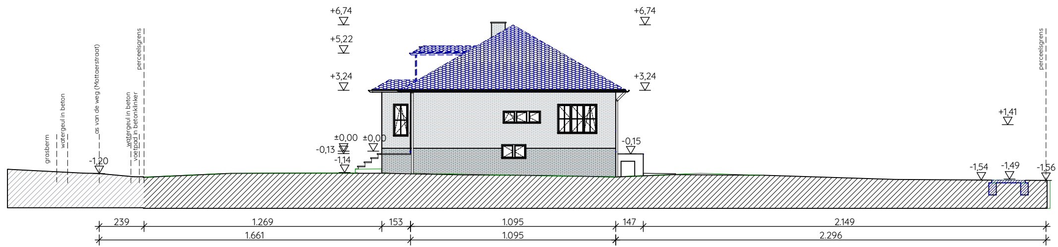
PROFIEL 2 bestaande toestand
