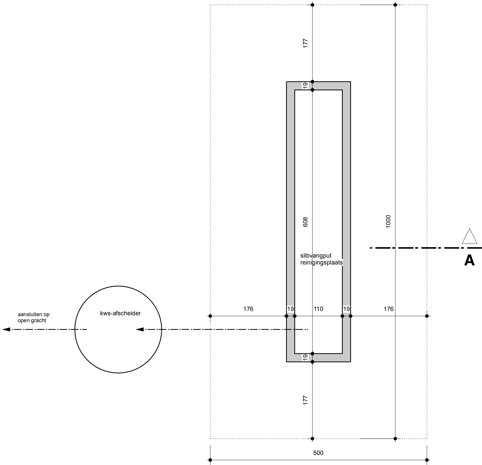
Funderingsplan _____reinigingsplaats landbouwvoertuigen
