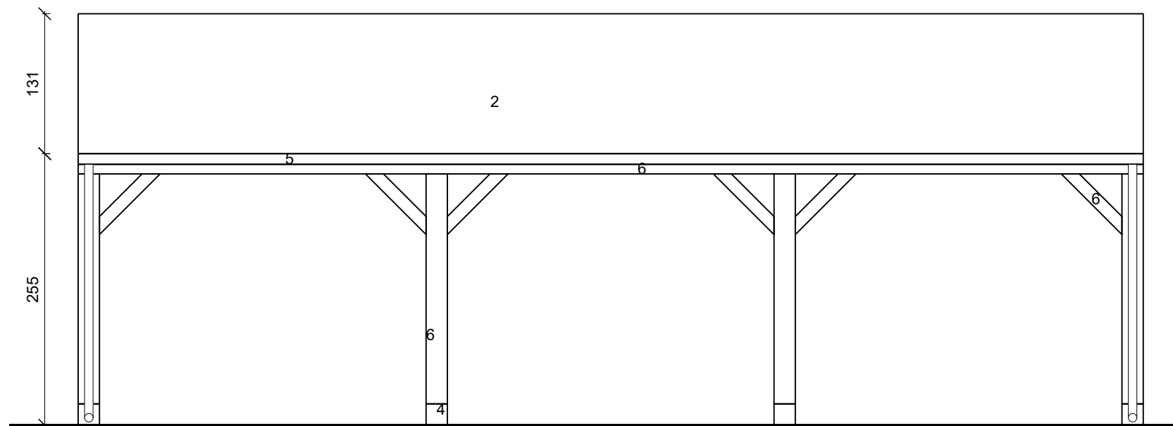
LINKER ZIJGEVEL
