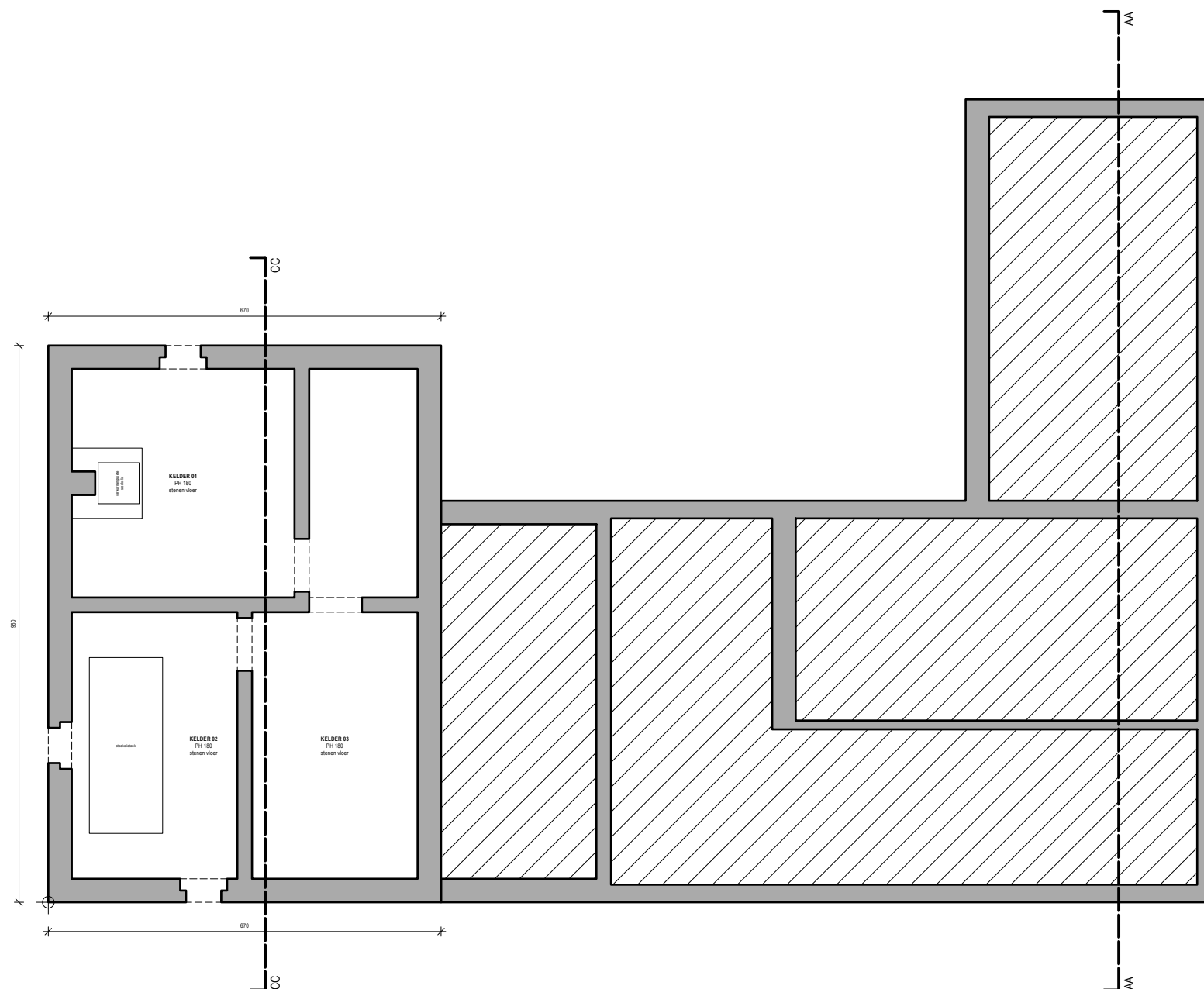
GRONDPLAN KELDER, FUNDERING EN RIOLERING BT
