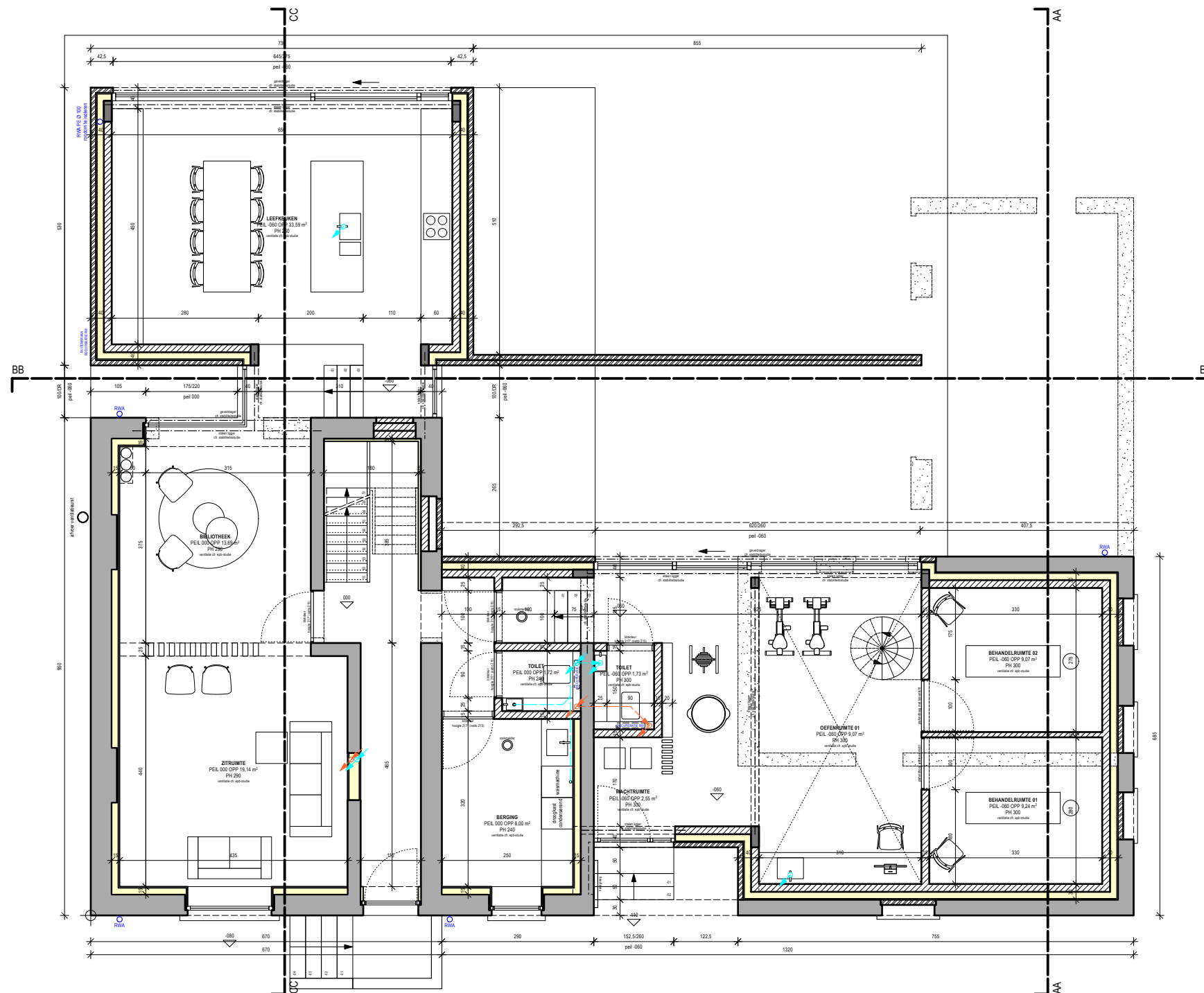
GRONDPLAN GELIJKVLOERS NT
