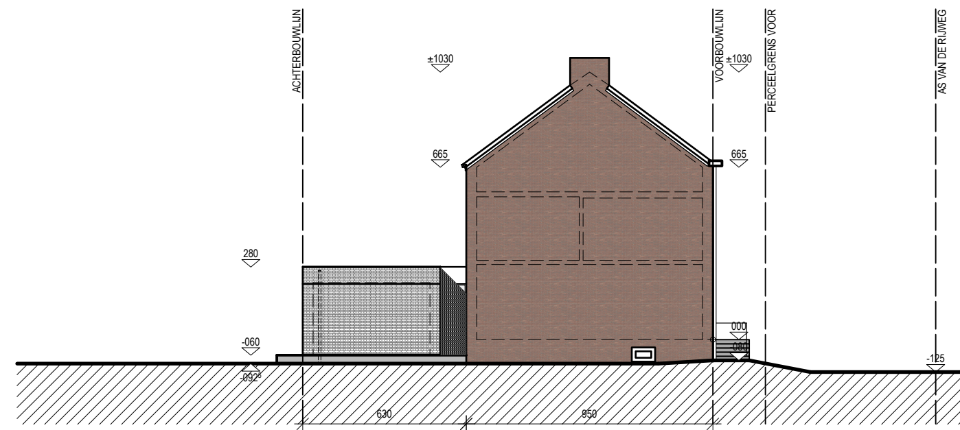
TERREINPROFIEL AA NT
