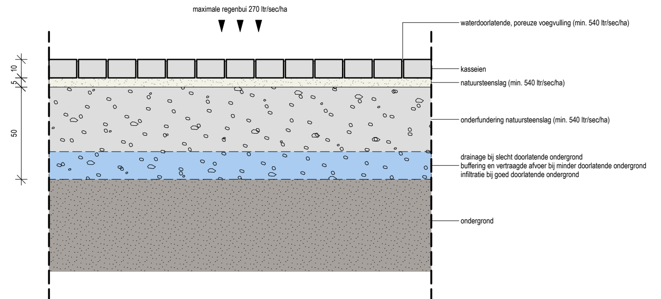
PRINCIPETEKENING WATERDOORLATENDE VERHARDING
