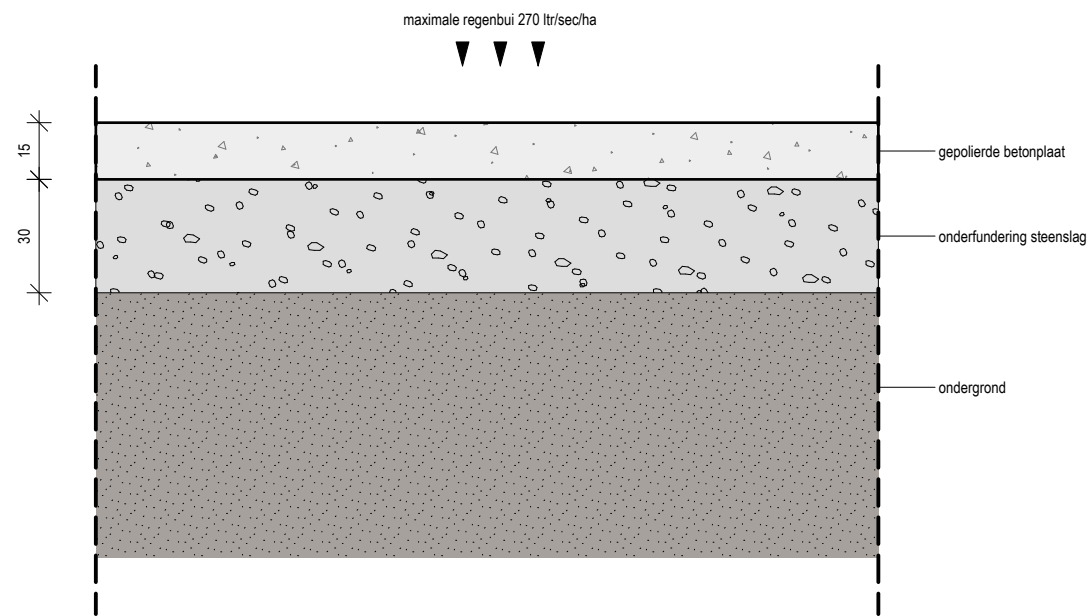
PRINCIPETEKENING NIET-WATERDOORLATENDE VERHARDING
